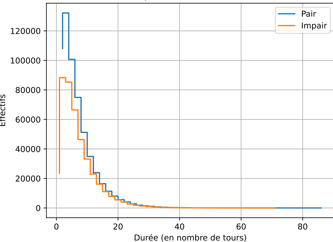
Durées de 1000000 de parties de bataille (4 couleurs de 3 cartes)
