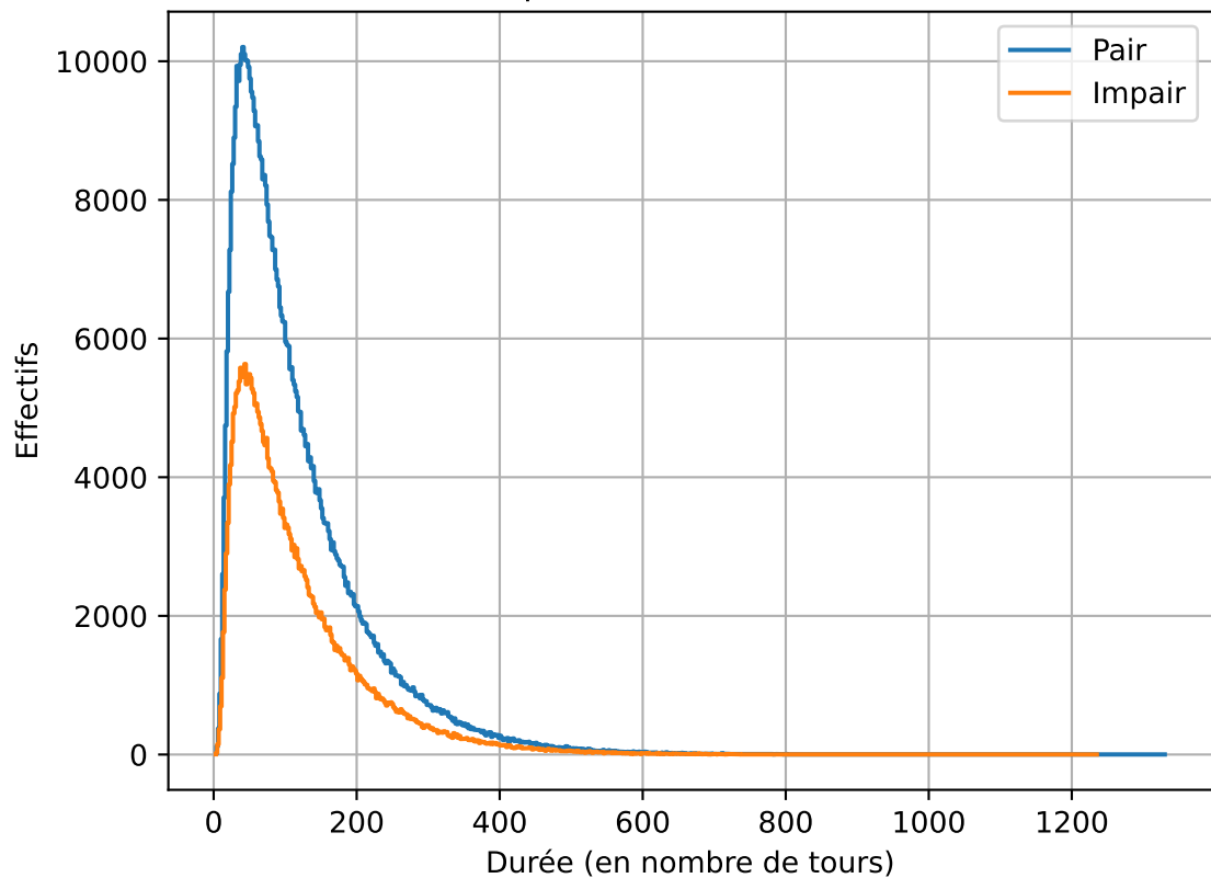
Durées de 1000000 de parties de bataille (8 couleurs de 5 cartes)
