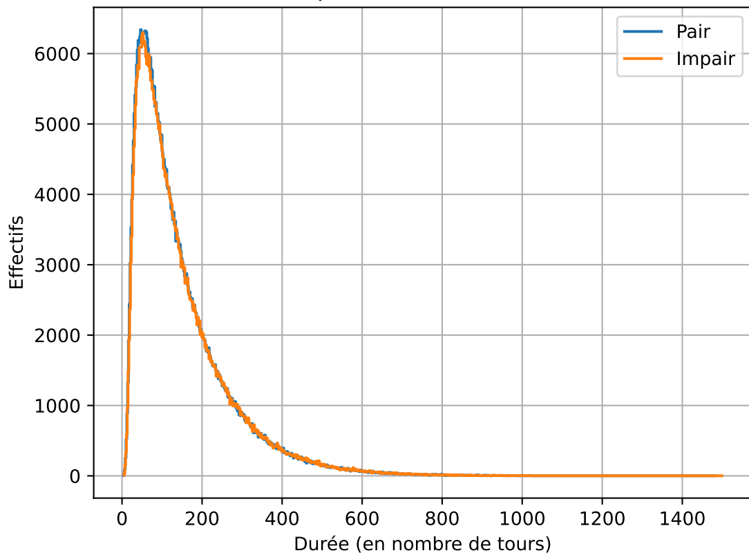
Durées de 1000000 de parties de bataille (9 couleurs de 5 cartes)
