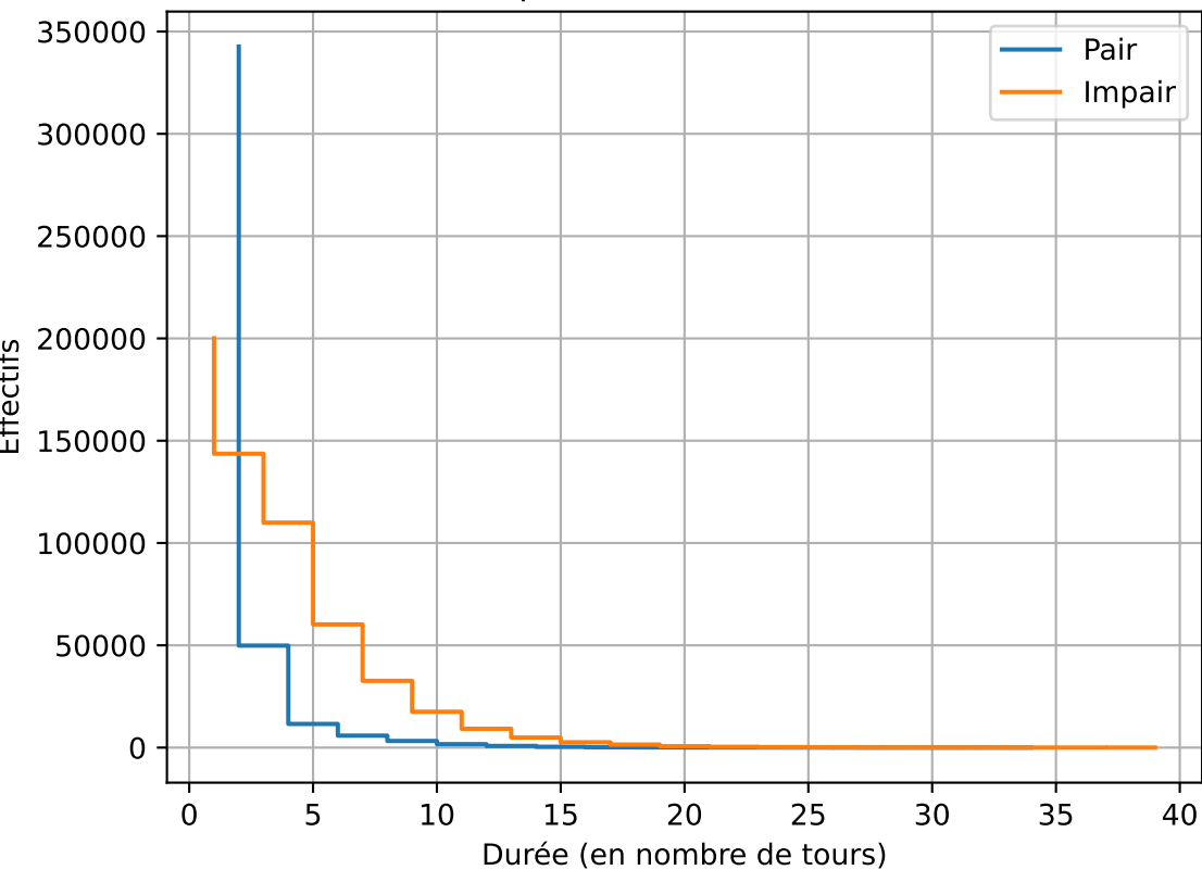
Durées de 1000000 de parties de bataille (4 couleurs de 2 cartes)
