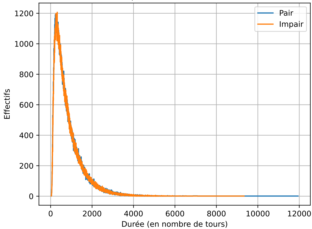
Durées de 1000000 de parties de bataille (9 couleurs de 9 cartes)
