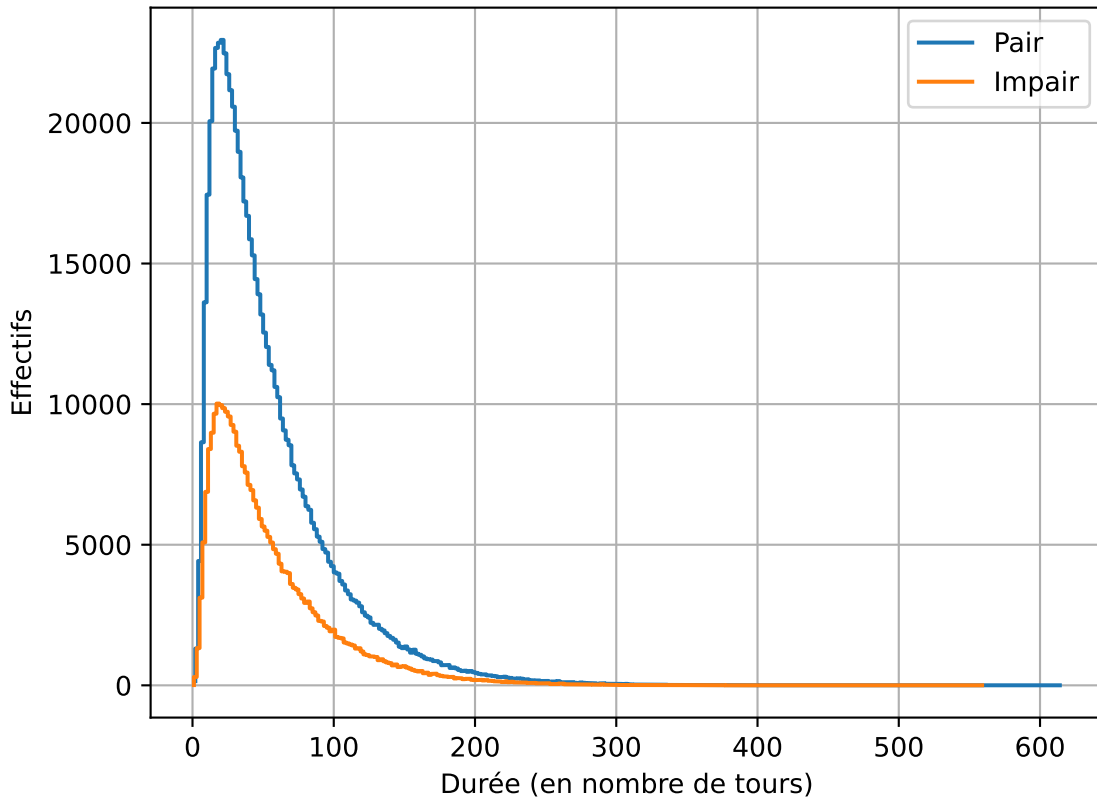
Durées de 1000000 de parties de bataille (4 couleurs de 6 cartes)
