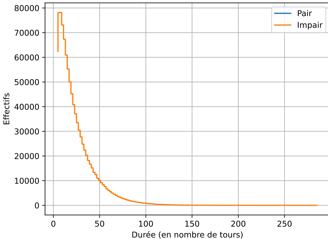
Durées de 1000000 de parties de bataille (1 couleurs de 10 cartes)
