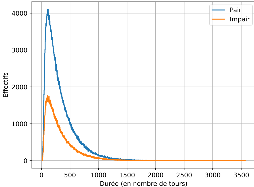
Durées de 1000000 de parties de bataille (8 couleurs de 7 cartes)
